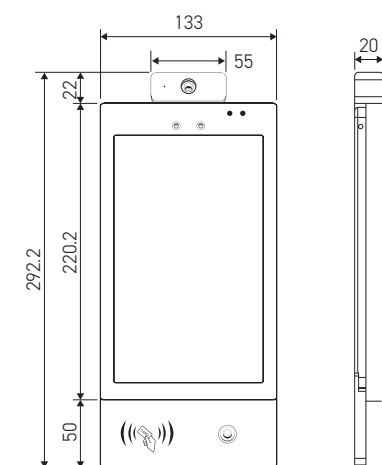
顔認証サーマルカメラ RF-01/RF-02
